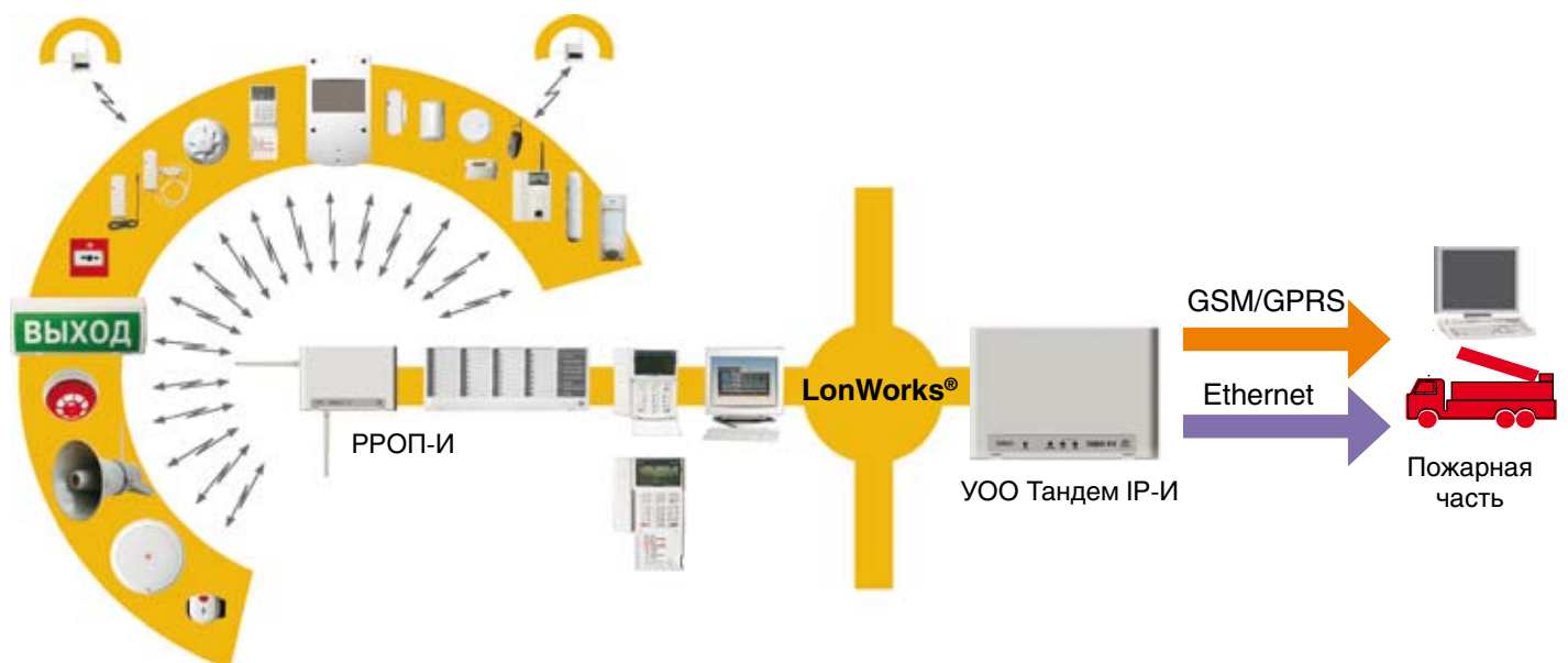
Рис.18. Пример подключения по протоколу LON (ИСБ «Стрелец-Интеграл»)
