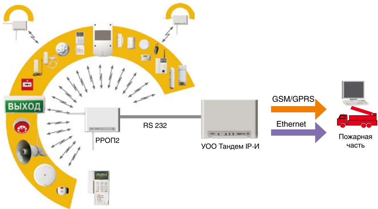
Рис.17. Пример подключения по протоколу RS-232 (ВОРС «Стрелец»)
