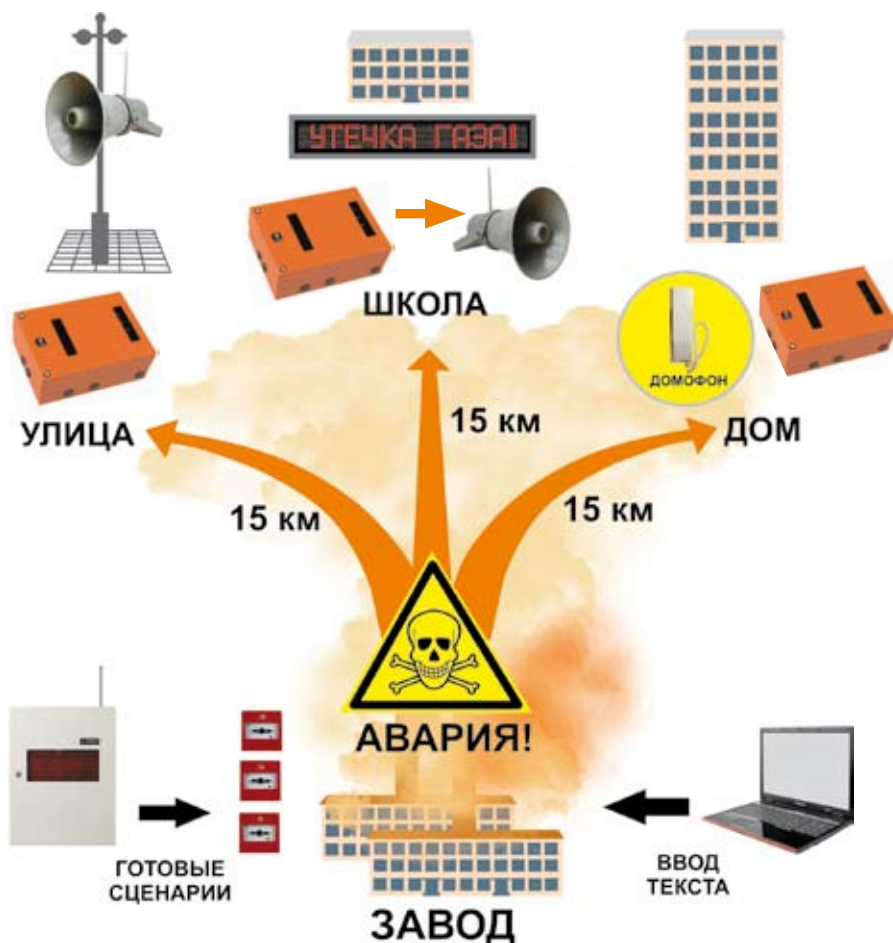
Рис.35. Объект «Территория»
